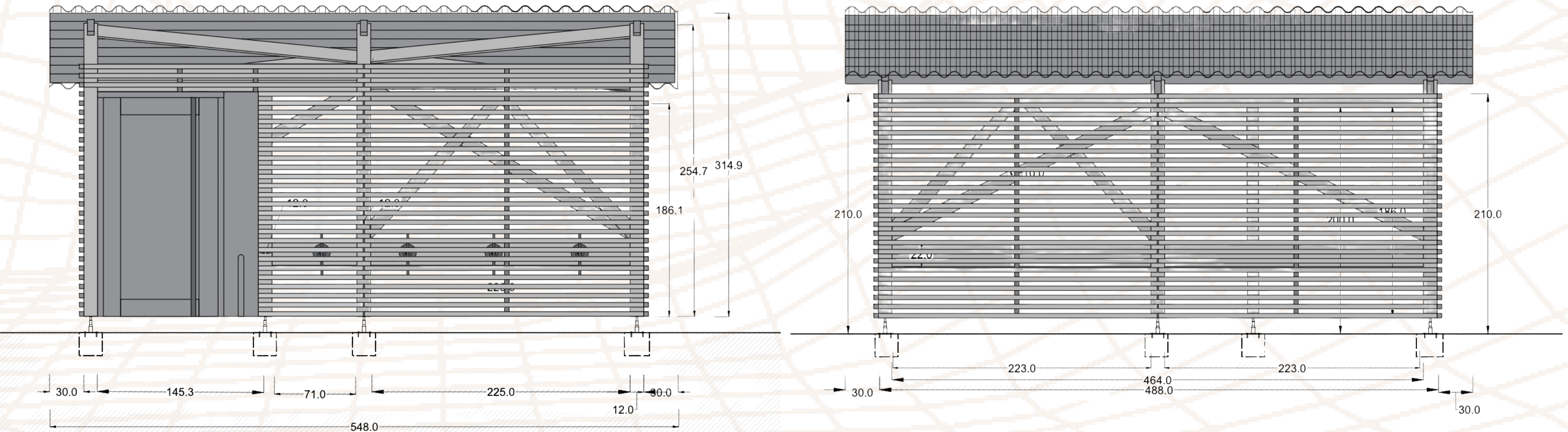
Façade D
